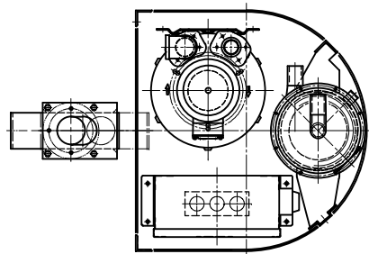
Cross section A-A A-A 断面
